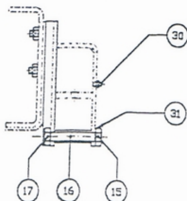
CORTE A A ESCALA 1:5
