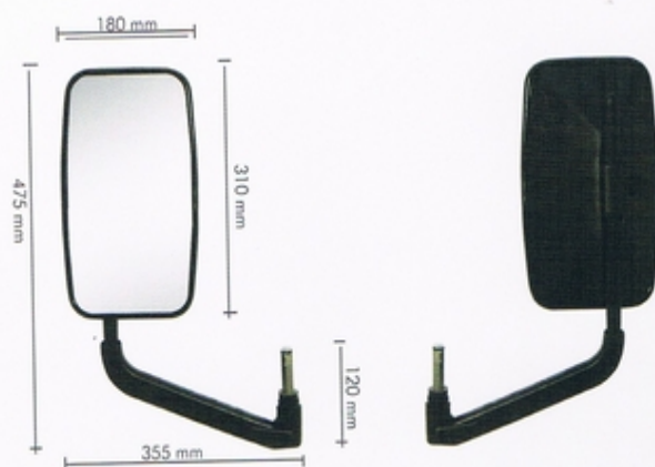
M-038F - Espelho Completo Original
