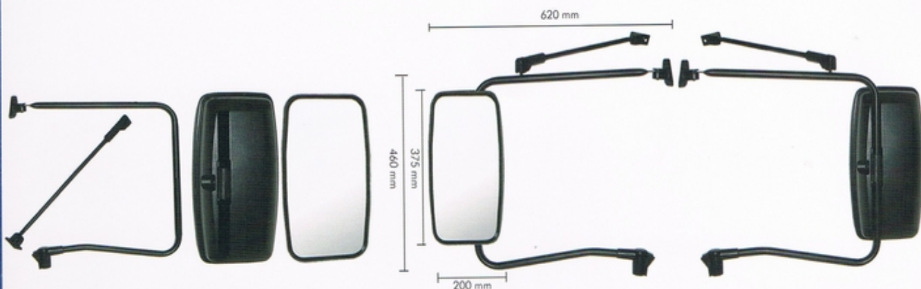
W-904 - Espelho Completo
