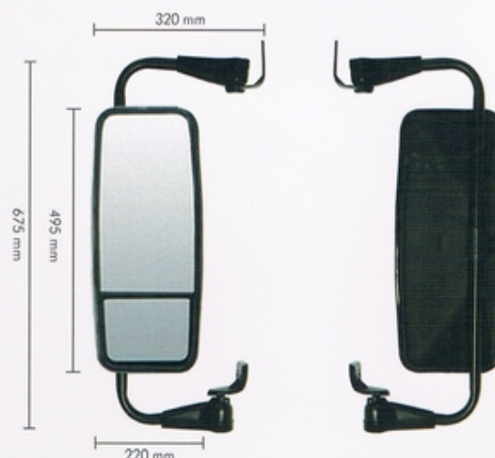
S-236 - Espelho Completo
