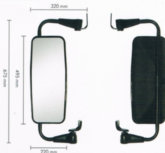
S-242 - Espelho Completo
