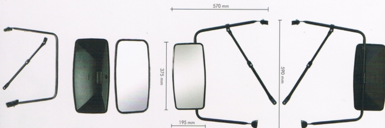
M-044J - Suporte (16mm) M-040 - Tirante (16mm)
