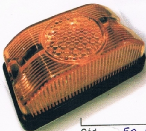
Cód. FO 530 Farol 1 polo ( bayoneta ) con reflector de acero inoxidable junta de goma (107 x 59 mm)
