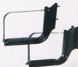
M-196U - Sup. Traseiro c/ Cinta M-196T - Sup. Dianteiro c/ Cinta M-023E - Cinta de Tanque
